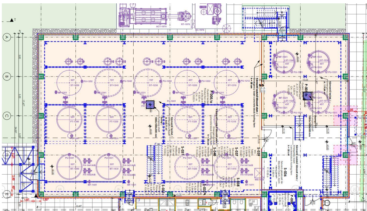
9. ábra: Belső Tartálypark
